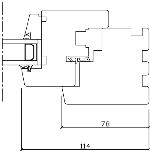
SNITT A-A
