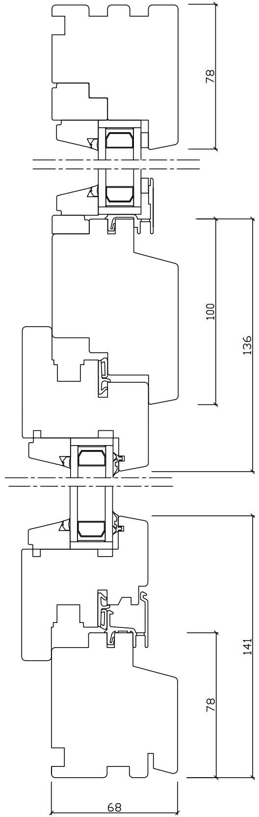
SNITT B-B
